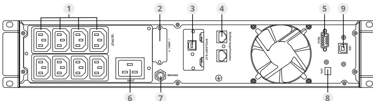
Рис. 2-3: Вид сзади: ИБП ИМПУЛЬС ФРИСТАЙЛ 2000 ВА
