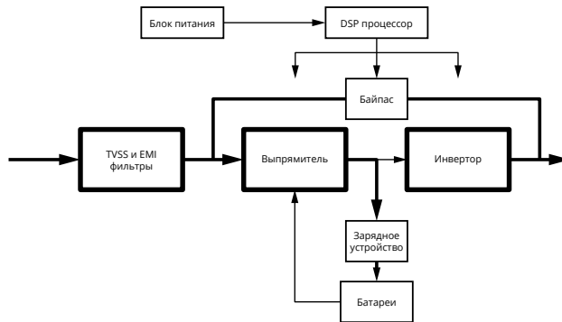
Рис 2-7: Режим байпаса
