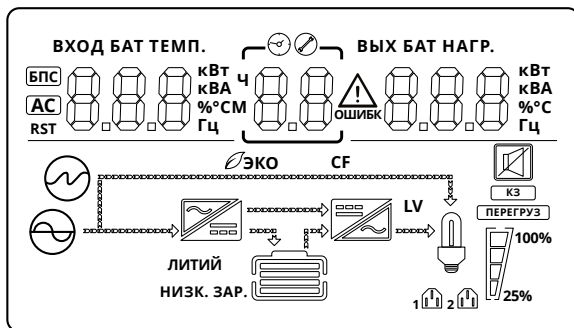
Рис. 4-2: ЖК-дисплей
