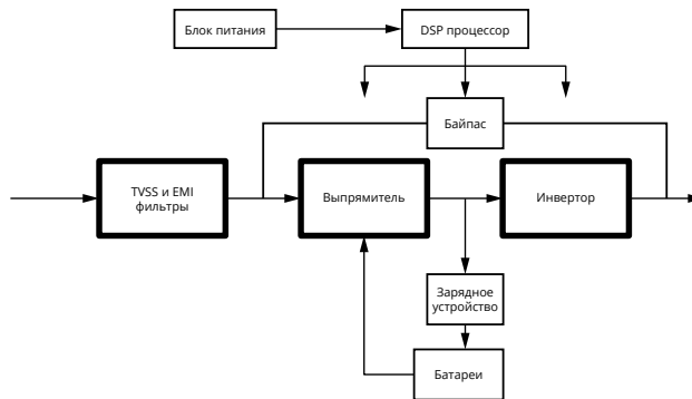
Рис 2-5: Система ИБП
